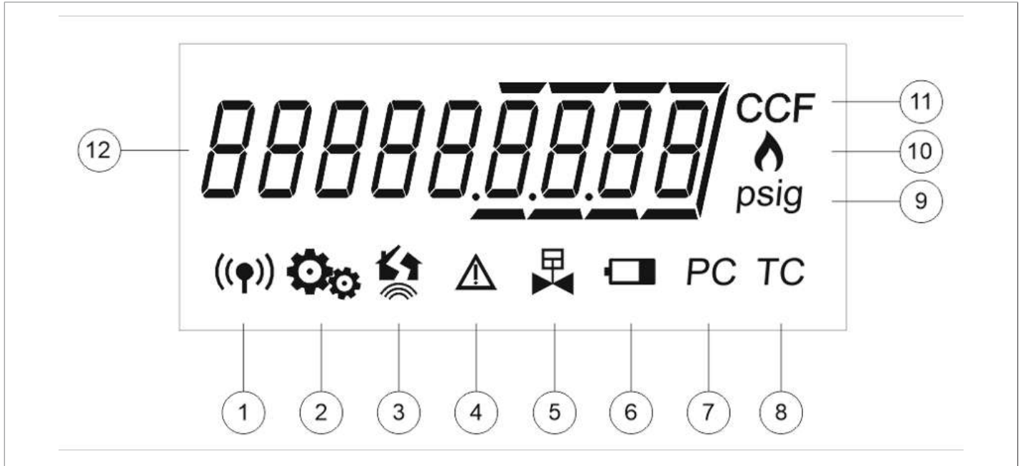
Fig. 5.4. LCD display SSM-ICON 250
